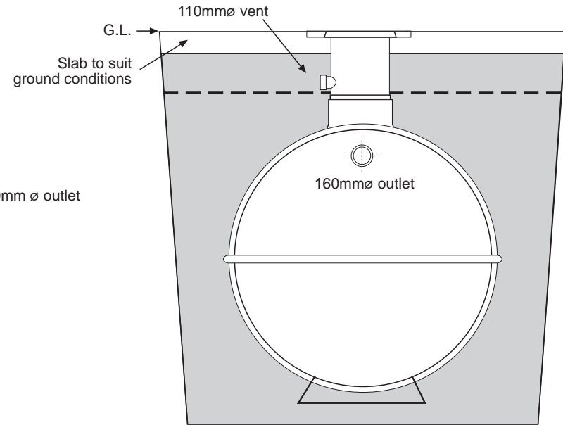
End elevation
